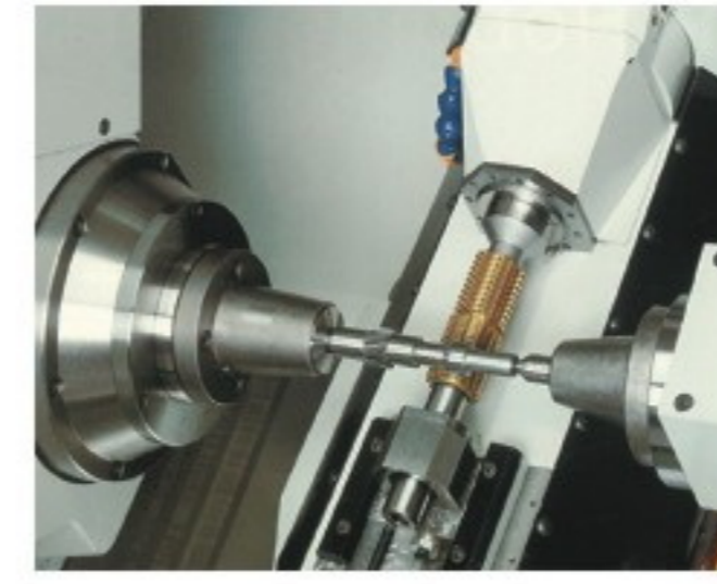
齒軸仿齒加工 PINION SKIVING
