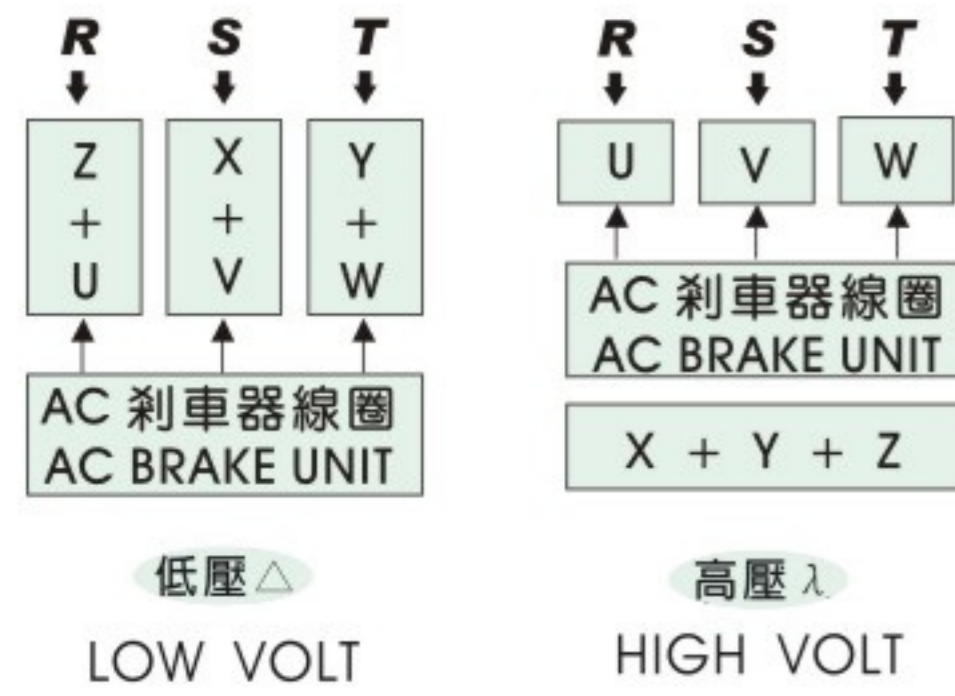
(c) 三相六條馬達電源線附交流剎車器 (SIX WIRES W/ AC BRAKE UNIT)
